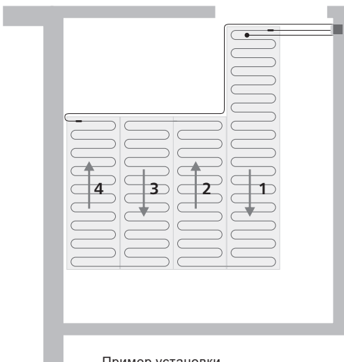
Пример установки нагревательной плёнки в кухне
