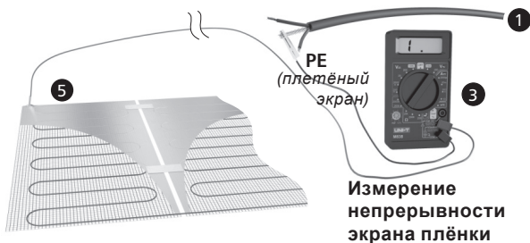
Измерение сопротивления изоляции плёнки
